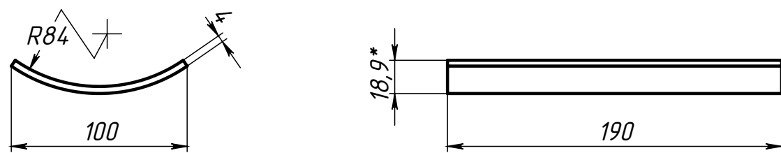
Поз.3 (Ложемент)
