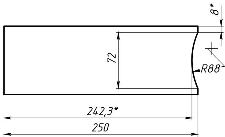
Поз.1 (Основание)
